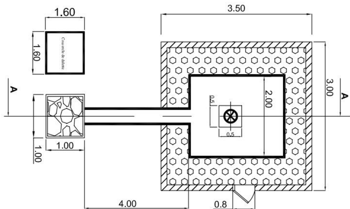
VUE DU PLAN D'AMENAGEMENT DE L'OUVRAGE
